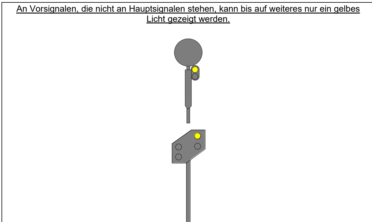
Signal Vr 1 -Fahrt erwarten-
