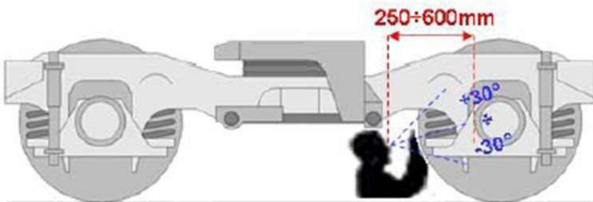
Abbildung 2-Inspektionswinkel und -abstand
