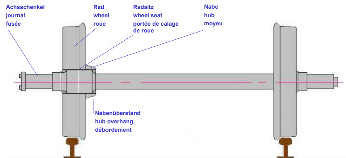
Radsatz
