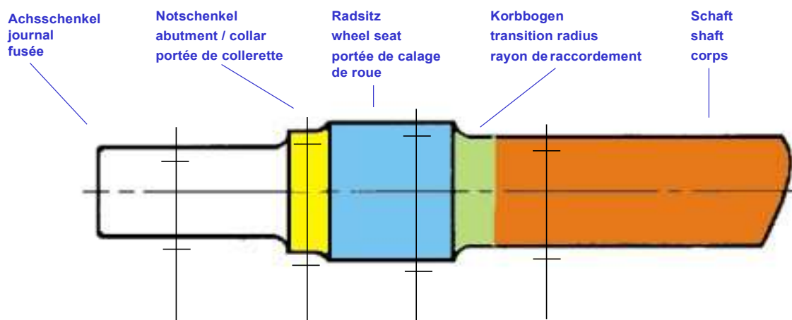
Radsatzwelle
