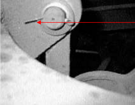
Bild 1 Abgescherter Splint
