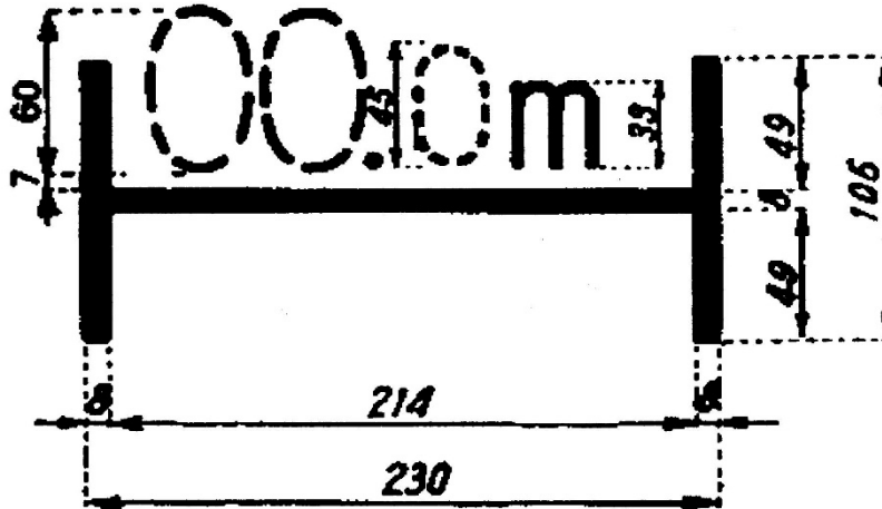
Bild 1 Ladelänge
